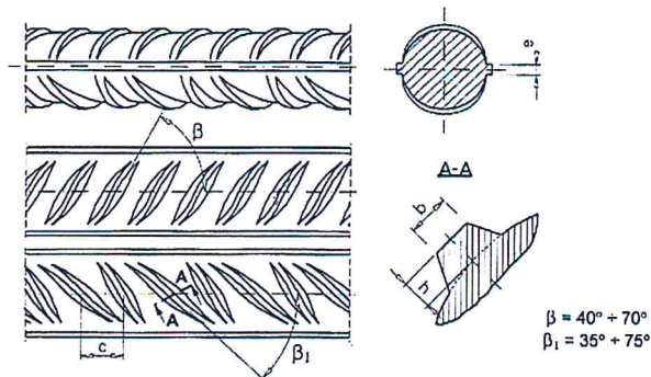
Obr. 1: Tvar a rozmístění žebírek oceli typ B500B
